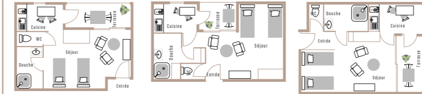
APPARTEMENT T1 DE 28,5 M 2 + TERRASSE
